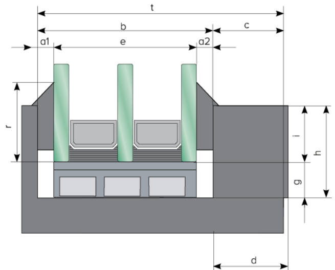
Abb. 2: Schematische Darstellung Glasfalz in Anlehnung an DIN 18545:2015-07 und DIN 52460:2015-12
