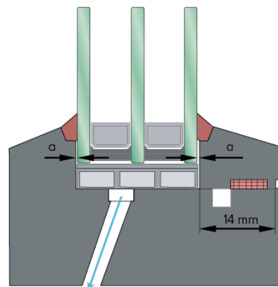
Abb. 3: Verglasung ohne Vorlegeband, Abstand „a“ ca. 0,5 mm bis 1,0 mm
