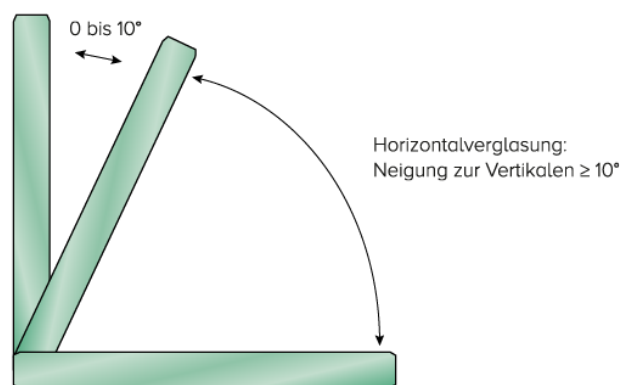
Abb. 4: Definition von Horizontalverglasung nach DIN 18008 (Nach der EN 13830 werden Horizontal- zu Vertikalverglasungen bei 15° unterschieden)
