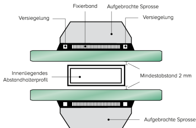
Abb. 5: Beispiel für Wiener Sprosse
